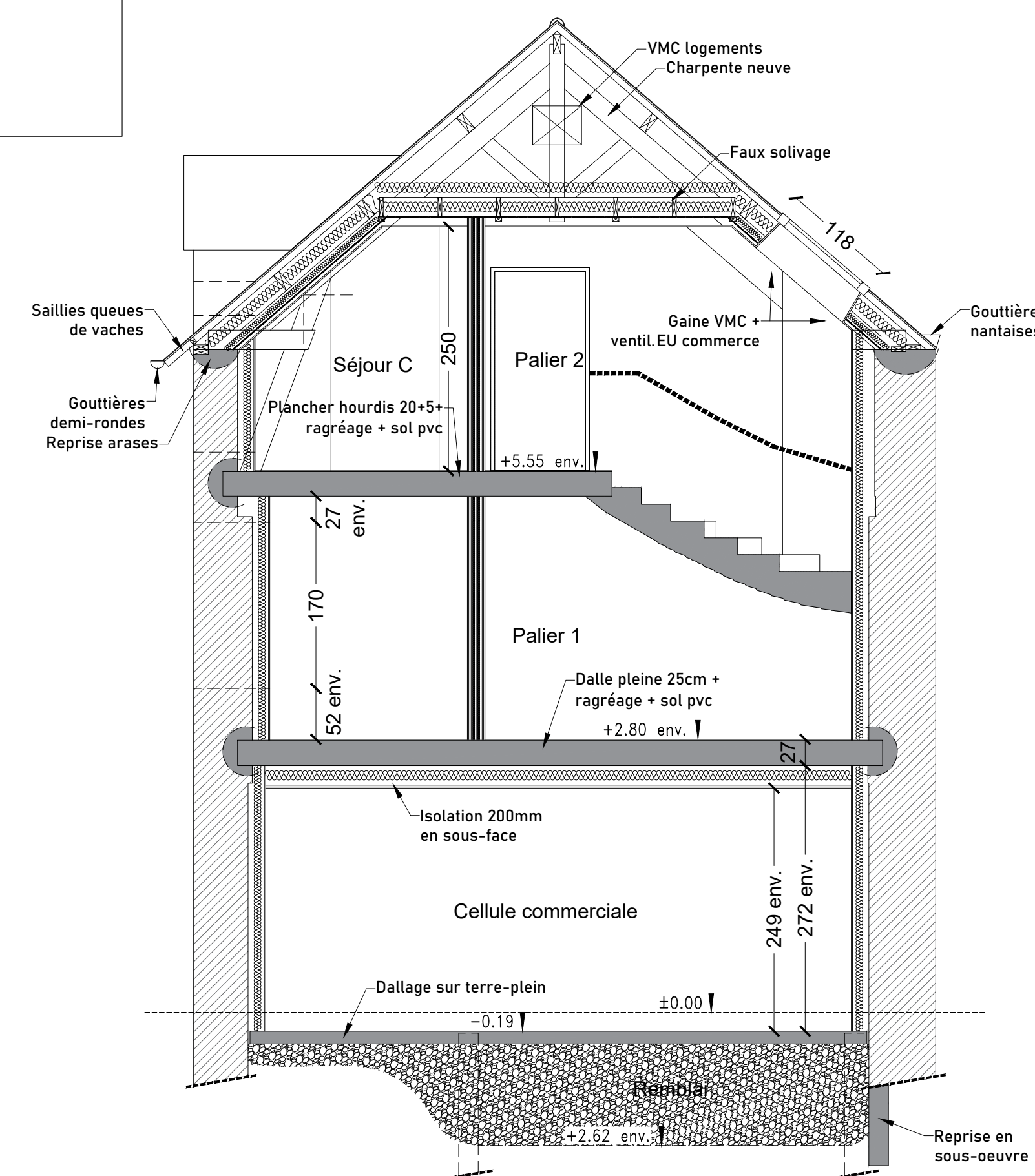
COUPE C-C
