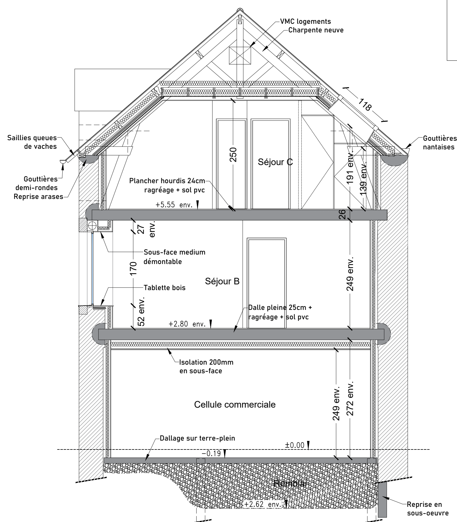
COUPE A-A
