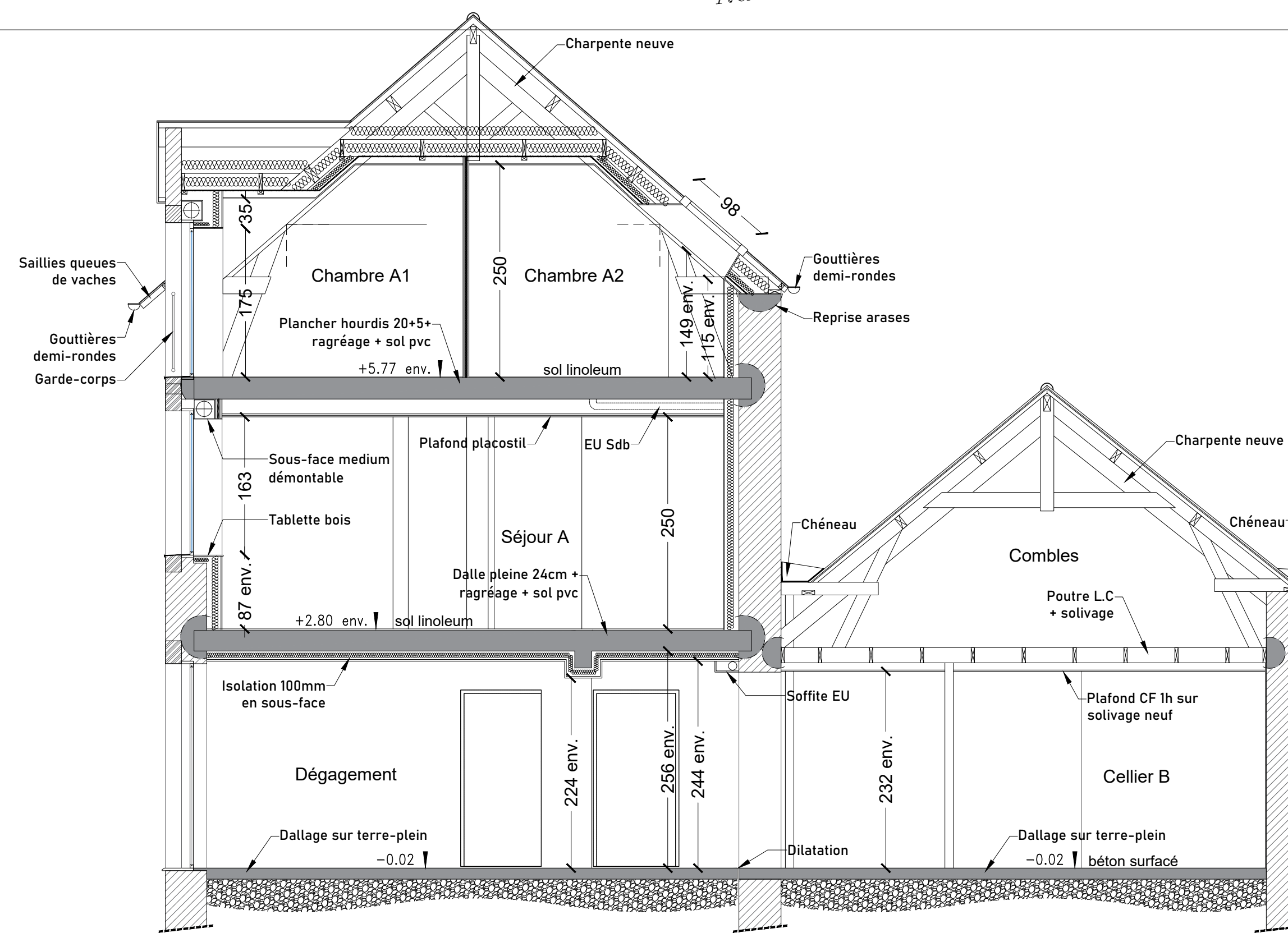
COUPE B-B
