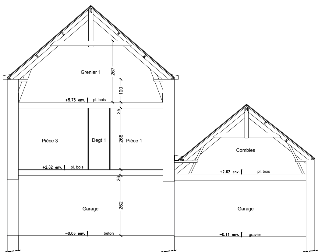
COUPE B-B
