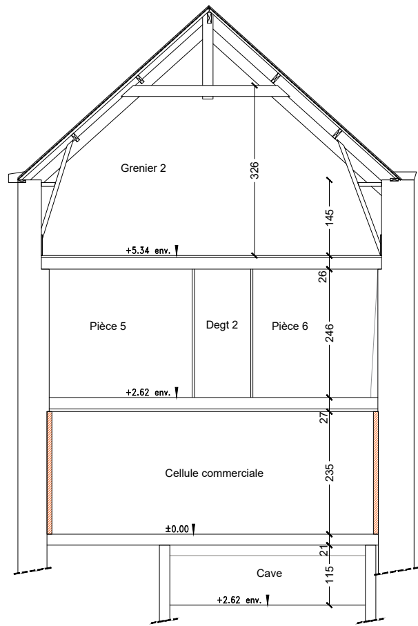
COUPE A-A
